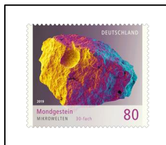
Mondgestein in 30-facher Vergrößerung
